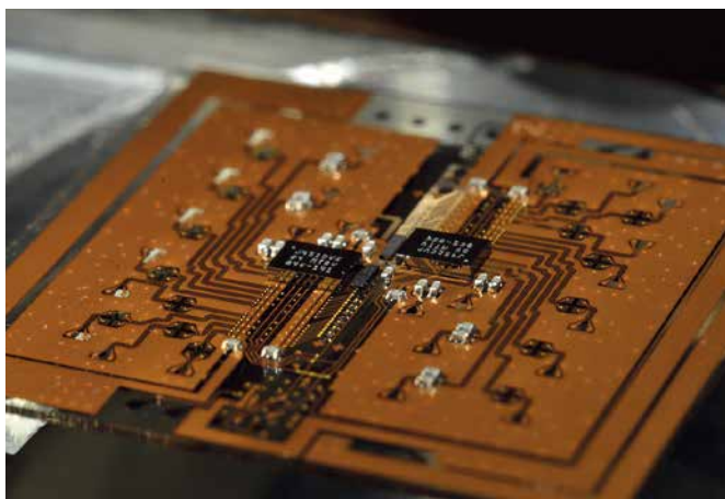
On-Board-Transceiver mit 4x25 Gbit/s/kanal auf Glasinterposer mit Durchkontaktierungen und integrierten Linsenarrays © Fraunhofer IZM
