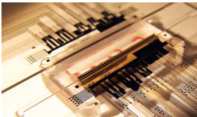
Umlenk-Spiegeleinheit zur optischen Ankopplung an einen mit elektrischen und optischen Wellenleitern versehenen Glas-Chip für EOCB/Backplane-Anwendungen © Fraunhofer IZM
