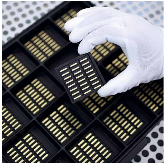
Diodenlaserbarren der Jenoptik Diode Lab GmbH © Jenoptik AG/Heiner Mueller-Elsner
