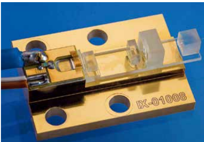
Vollständig glasbasierte mikro-optische Bank für kompakte Diodenlasermodule mit Strahldrehung und Zusammenführung mehrerer Kanäle auf eine optische Faser © Fraunhofer IZM
